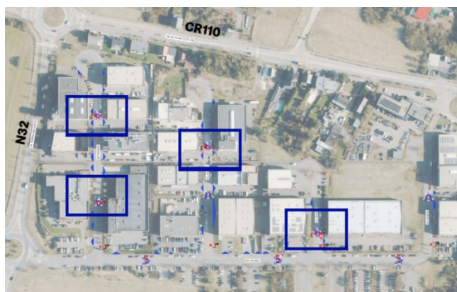
Pose d'un coussin berlinois à 30km/h et rétrécissement de la chaussée
