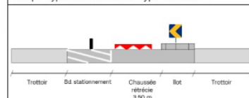
Coupe-type: ralentisseurs du type « coussin »
